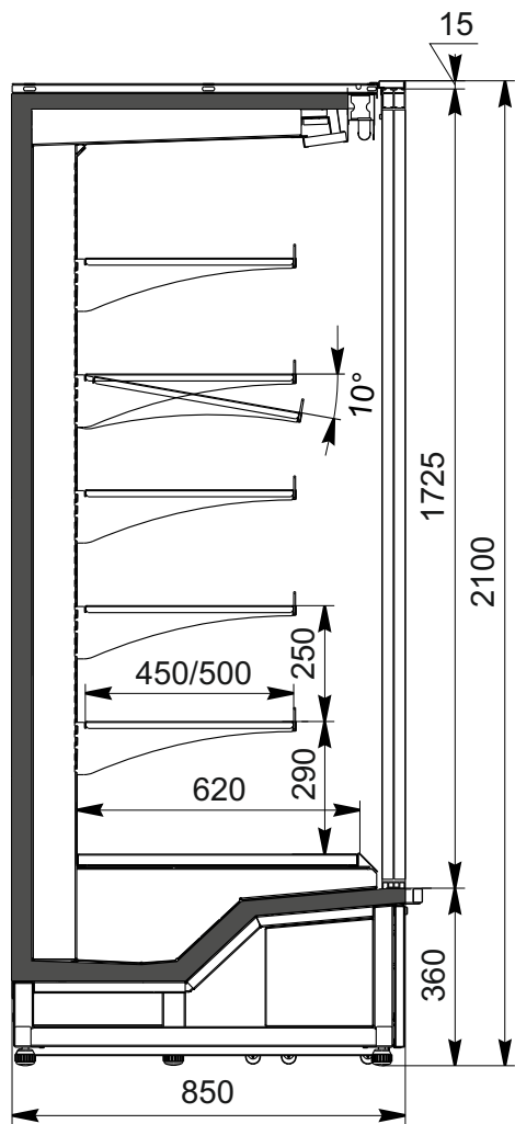
Indiana medium AV 085 MT D 210-DLM
