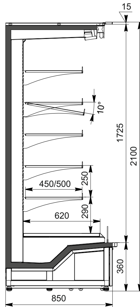
Indiana medium AV 085 MT O 210-DLM
